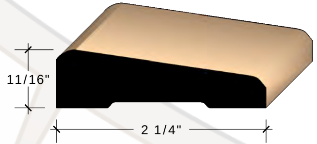
11/16" X 2 1/4" BEVEL CASING FINGERJOINT PINE/MDF More info
