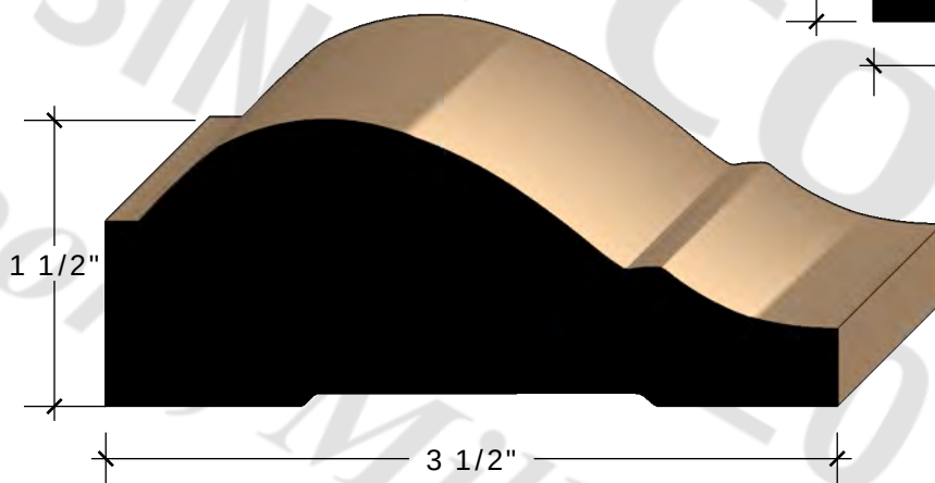
1 1/2" X 3 1/2" BIG FOG CASING FINGERJOINT PINE
