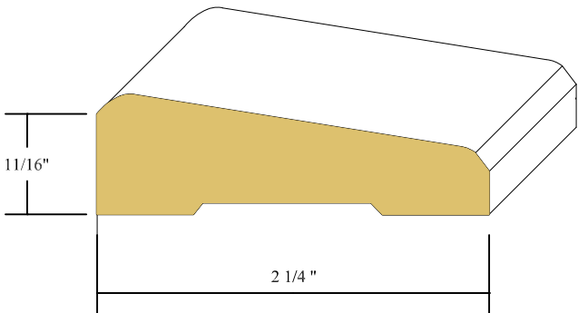
11/16" X 2 1/4" BEVEL CASING FINGERJOINT PINE
