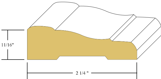
11/16" X 2 1/4" M/E CASING FINGERJOINT PINE
