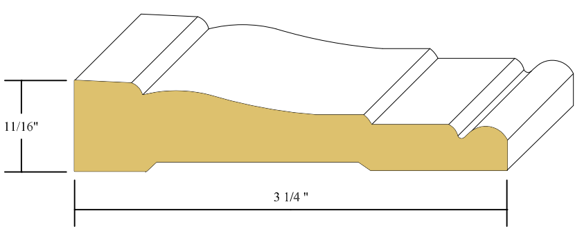
11/16" x 3 1/4" M/E CASING FINGERJOINT PINE
