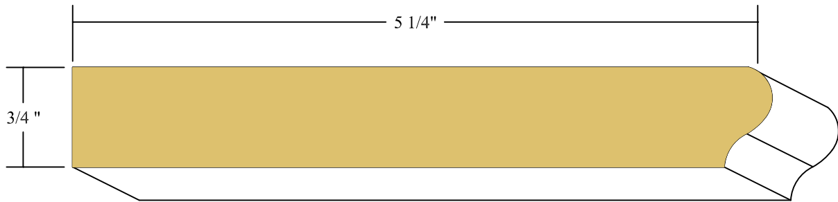
11/16" X 5 1/4" FLAT STOOL FINGERJOINT PINE/MDF
