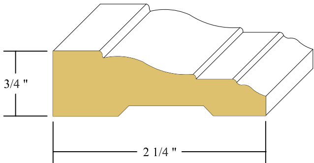
11/16" X 2 1/4" 366 CASING FINGERJOINT PINE
