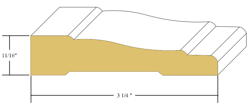
11/16" x 3 1/4" M/E CASING FINGERJOINT PINE
