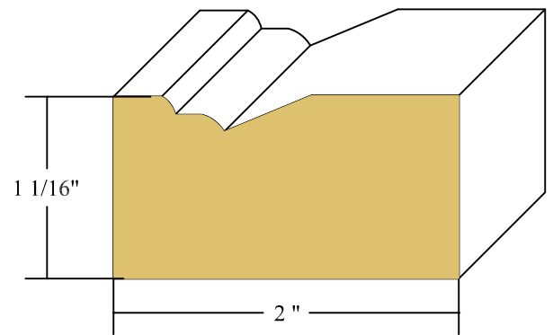
1 1/16" X 2" KOLBE BRICK MOULD FINGERJOINT PINE/PVC
